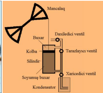
1784-cü il, Ceyms Uatt tərəfindən ixtira olunan buxar maşını və onun iş prinsipi
